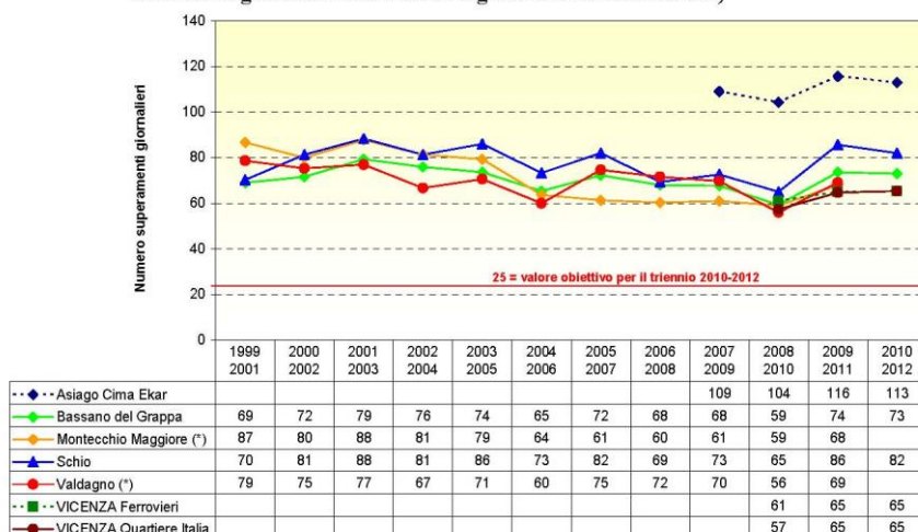
Medie triennali dei superamenti giornalieri del valore di 120 \mu\text{g}/\text{m}^3 da parte della massima media mobile 8 ore, intervallo 1° aprile – 30 settembre (valore obiettivo uguale a 25 secondo D. Lgs. n. 155 del 13/08/2010)
