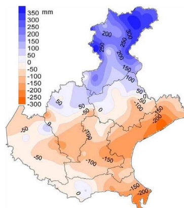
Precipitazioni 2012 differenze (mm) rispetto alla media del periodo 1992-2011
