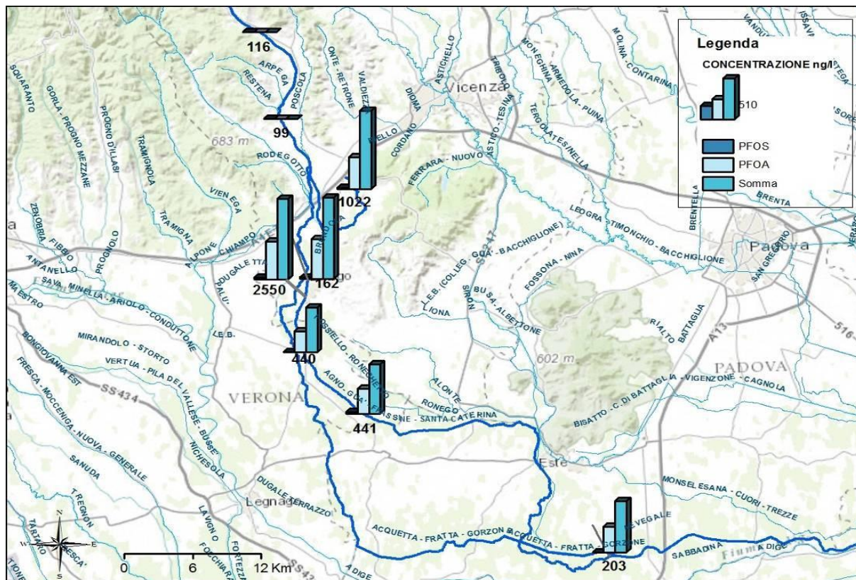
Campagna di Marzo 2014. Rappresentazione concentrazioni PFOS, PFOA e PFAS (ng/l) lungo il corso d'acqua Brendola-Guà-Frassine-Santa Caterina
