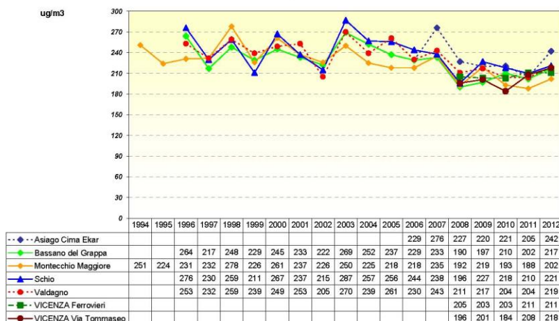
Massimi valori orari, intervallo aprile-settembre (aprile-luglio per le stazioni di Montecchio Maggiore e Valdagno)
