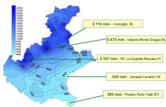
Precipitazioni in mm nel 2012 in Veneto
